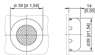
Pulsador luminoso 8602/3-735 Actuador con accionamiento axial
