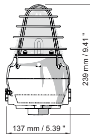
Baliza luminosa de destellos FX15
