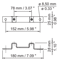
Soporte de fijación
