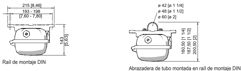
Rail de montaje DIN
