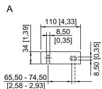
Escudra de fijación de pared montada en rail de montaje DIN
