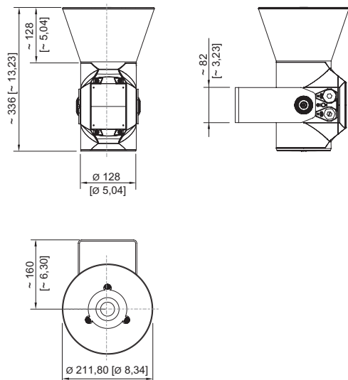
Bocina direccional YA60/3
