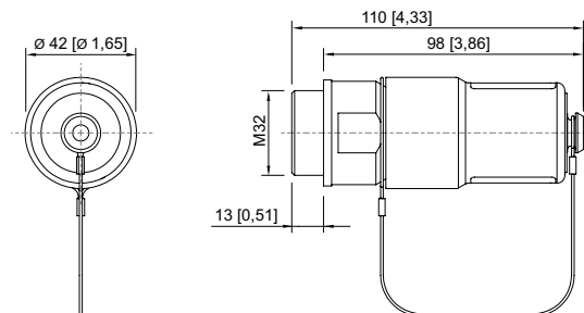
Base de brida Ex e 8595/1
