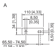
Escudra de fijación de pared montada en raíl de montaje DIN
