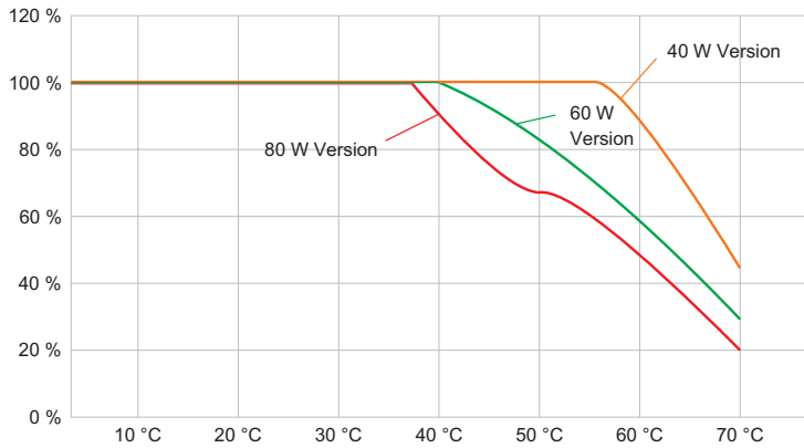
Depreciación luminosa con respecto a la temperatura ambiente - Variantes con DALI
