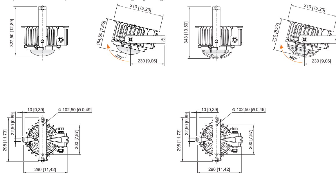
Con soporte de montaje
