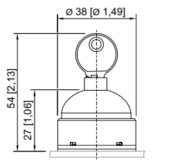
Interruptor de llave 8003/...-008
