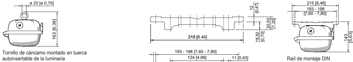
Rail de montaje DIN
