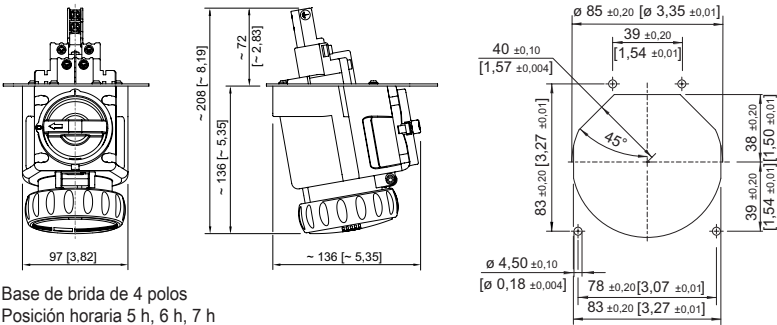
Base de brida de 4/5 polos Esquema de las aberturas
