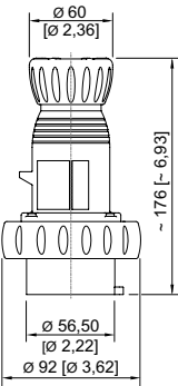
Enchufe de 5 polos
