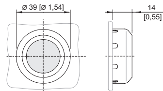
8602/3-001 Кнопочный выключатель Кнопочный переключатель с осевым управлением
