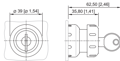
8602/3-006 Грибовидная западающая кнопка К/Ч 8602/3-009 Грибовидная западающая кнопка К/Ж Кнопочный переключатель с осевым управлением
